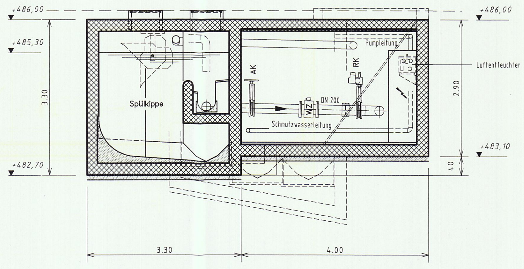
Schnitt C - C
